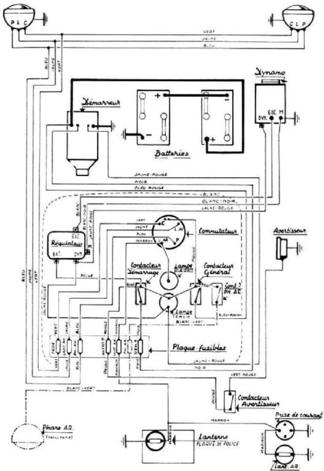
Fig. 42. - Circuit électrique.
