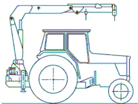
Gru per autocarro montata su trattore
