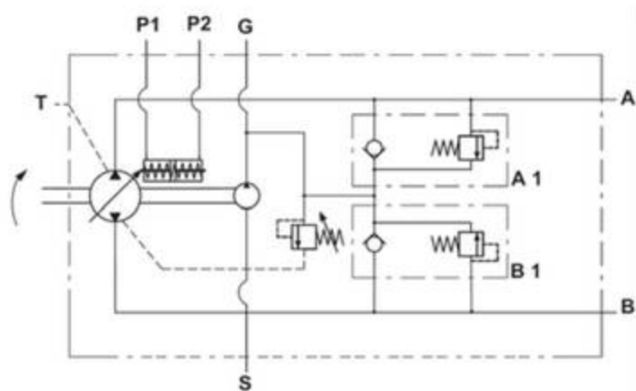
Schema idraulico
